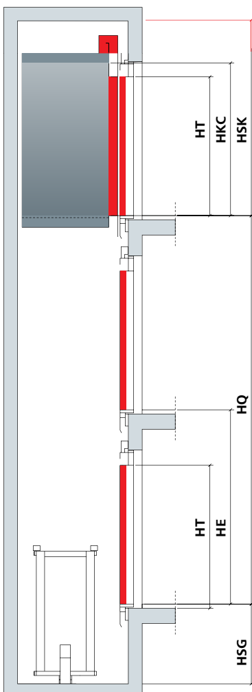
Einseitiger Zugang
